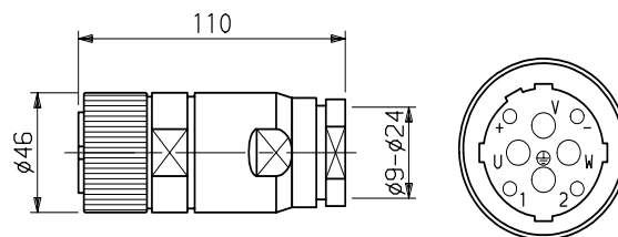
PLUG 220065R3610/3611
